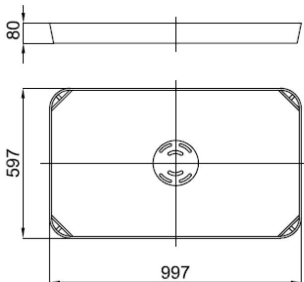
Rys. 1 Wymiary pokrywy PCZsB
