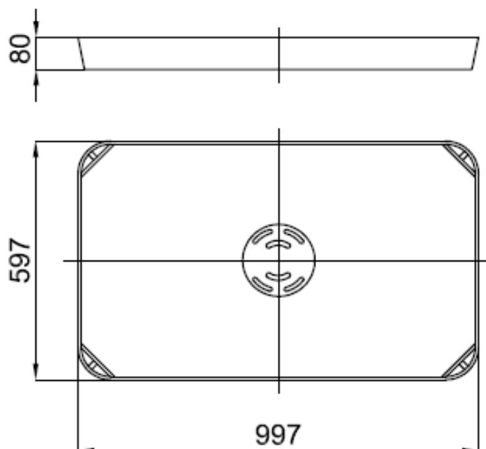
Rys. 1 Wymiary pokrywy PCZsD
