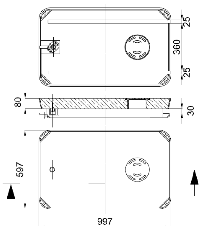
Rys. 1 Wymiary pokrywy PCZsBr
