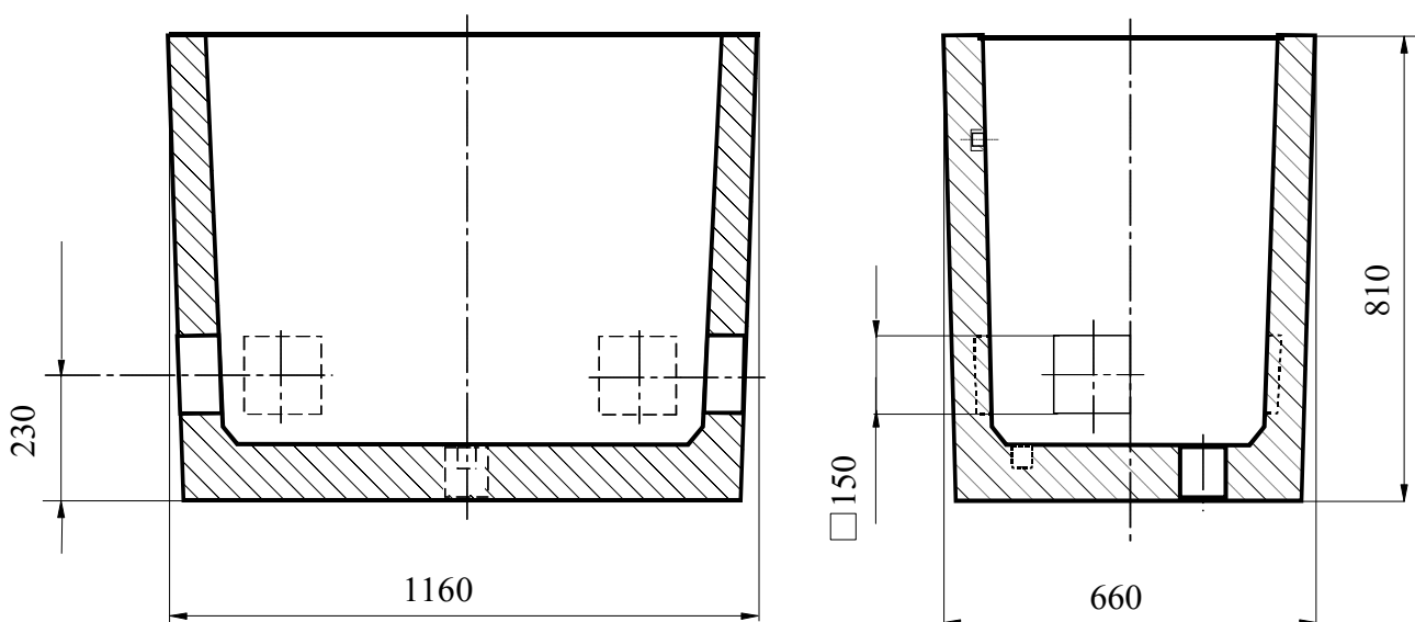
Rysunek 1. Wymiary studni kablowej SKR-1
